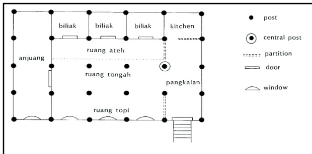
Gambar 10. Sirkulasi Udara Pada Rumah Gadang (Sumber: Analisa Penulis, 2012)
