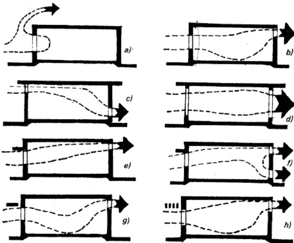
Gambar 3. Ventilasi Silang (horizontal) Hasil Penelitian dari Texas Engineering Experiment Station (Sumber: Mangunwijaya, 1988)
