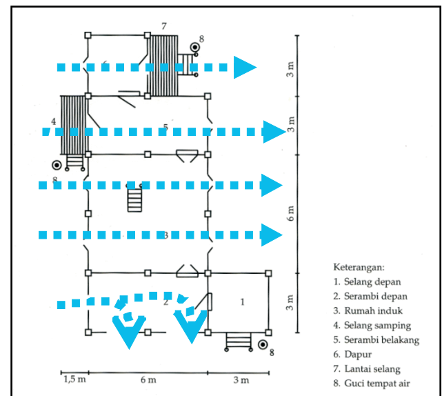
Gambar 14. Sirkulasi Udara pada Rumah Tradisional Melayu (Sumber: Analisa Penulis, 2012)
