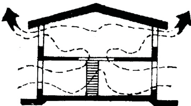
Gambar 4. Prinsip Ventilasi Vertikal (Sumber: Mangunwijaya, 1988)
